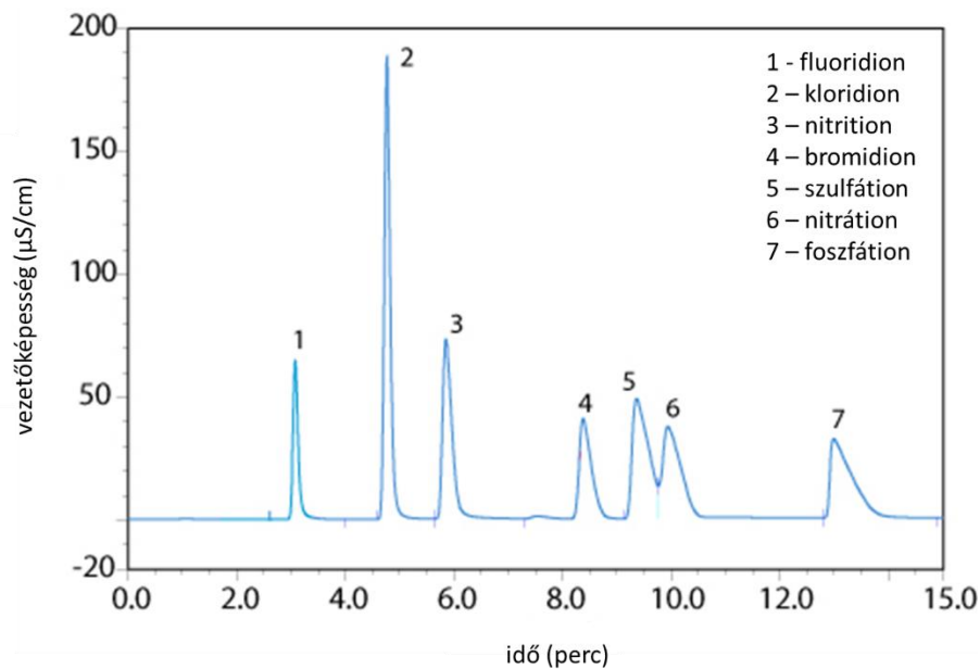
1. ábra: Egy tipikus anionkromatográfiai kromatogram
